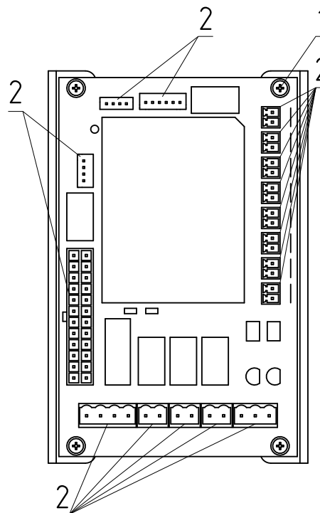
Рисунок 1. Блок управления
